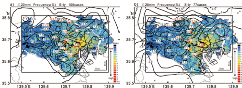
図2 東風時(a)と南風時(b)における1時間20mm以上の強雨頻度割合(%)。図の背景は50m四方の領域における最大の建築物階数の分布を表す(黄から赤になるほど階数が高い)。
