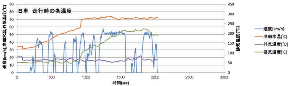
路上走行による A 車、B 車の NOx 排出濃度,各温度等
