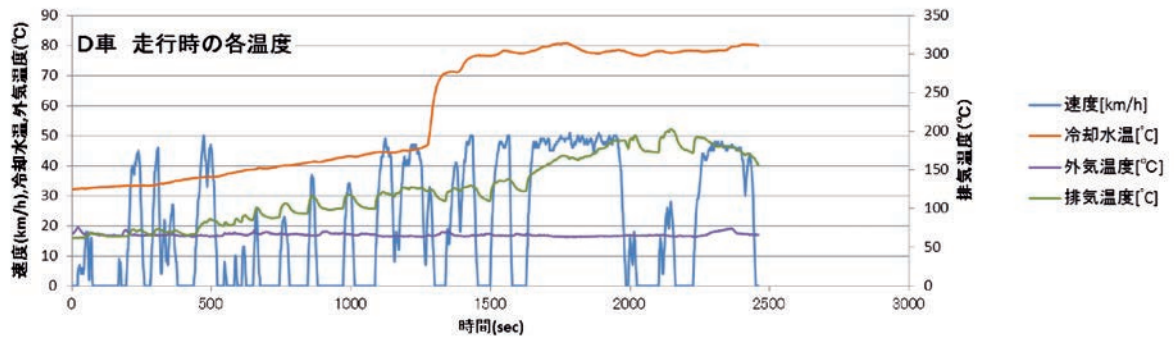
路上走行による C 車、D 車の NOx 排出濃度,各温度等
