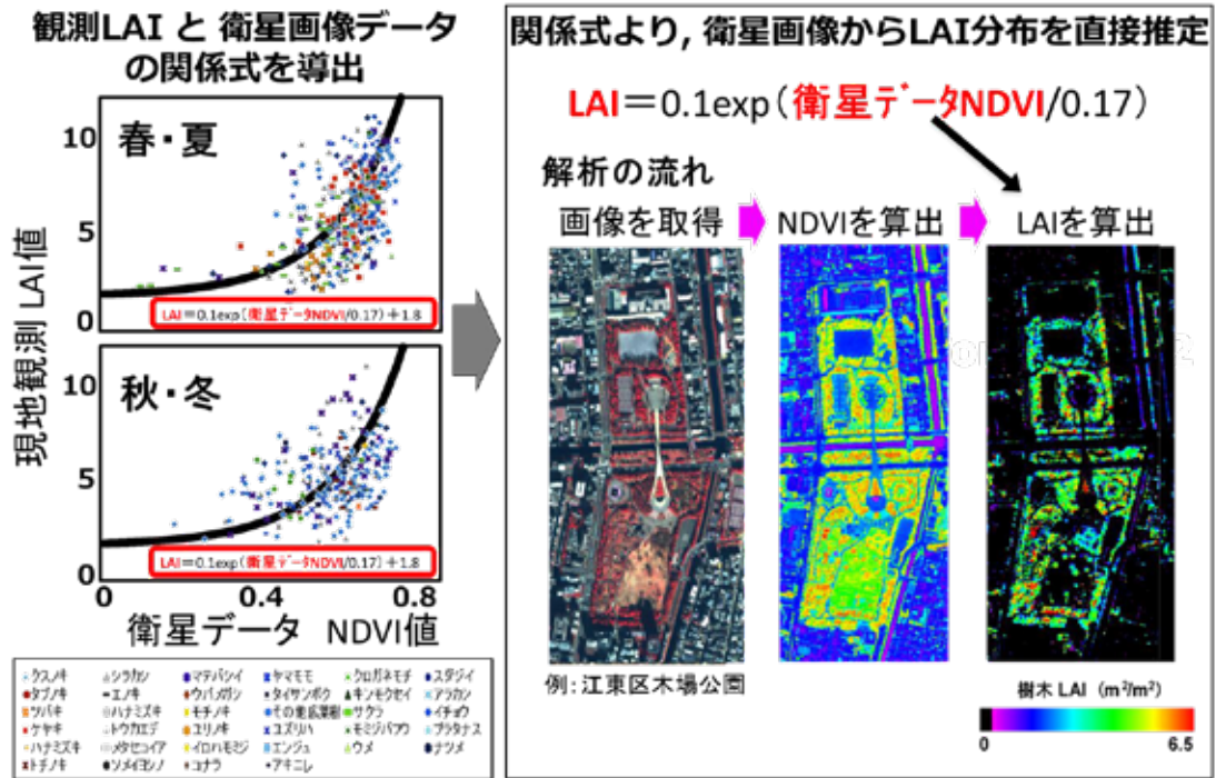
図 1. (左図) 導出した LAI-NDVI 関係式、(右図) その関係式を用いた樹木葉面積 (LAI) の推定方法
