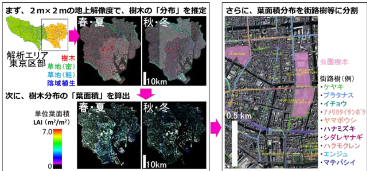
図 2. (左図) 東京区部の樹木葉面積分布の推定結果、(右図) 樹種別の街路樹・公園樹木への領域分割結果の例 分割領域以外に分布する樹木は「その他の樹木」とした
